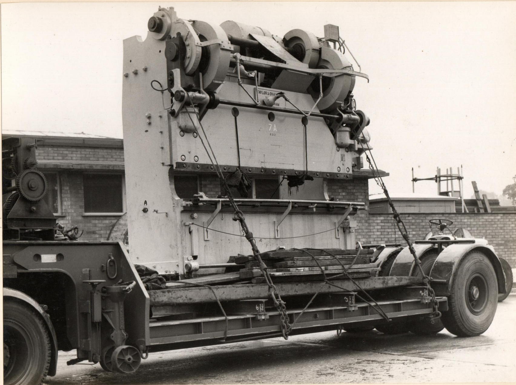
TAYLOR & CHALLENGER PRESS
